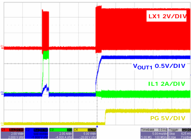
図 29. 出力短絡からの復帰、チャンネル 1
