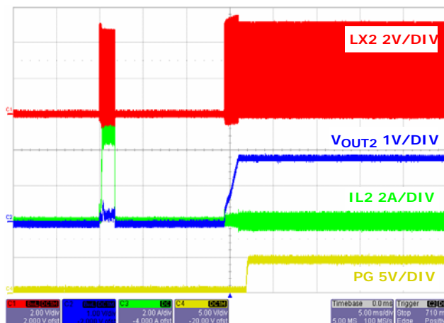
図 31. 出力短絡からの復帰、チャンネル 2
