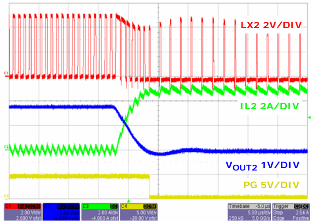
図 30. 出力短絡、チャンネル 2
